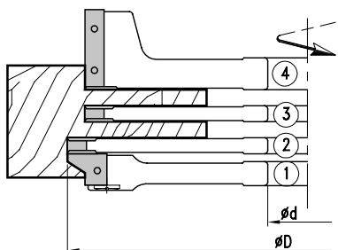
Wechselmesser/Ersatzteile Reversible knives/Spare parts
