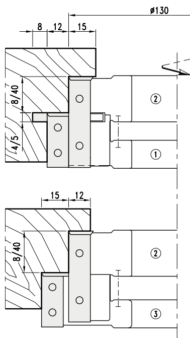
Wechselmesser/Ersatzteile Reversible knives/Spare parts
