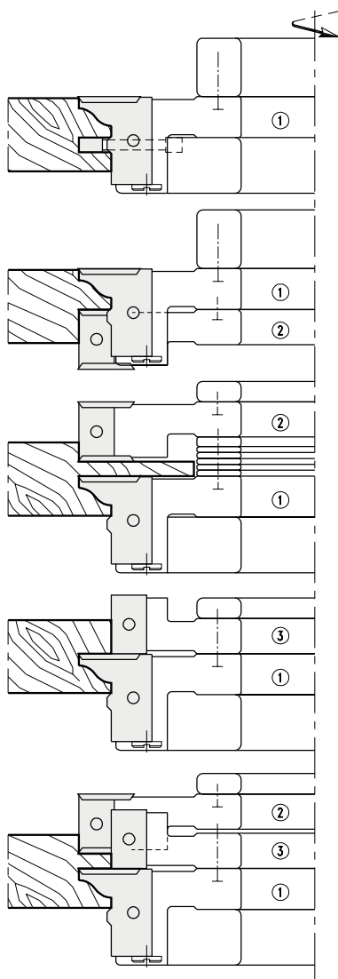
Wechselmesser/Ersatzteile Reversible knives/Spare parts
