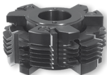
Radienprofil-Verleimfräser, verstellbar Softline gluejoint cutter, adjustable
