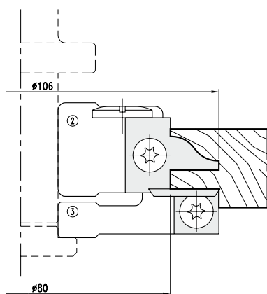
Wechselmesser/Ersatzteile Reversible knife/Spare parts
