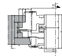
Vertikalflüster-Blendrahmen N78 Innenprofilierung
