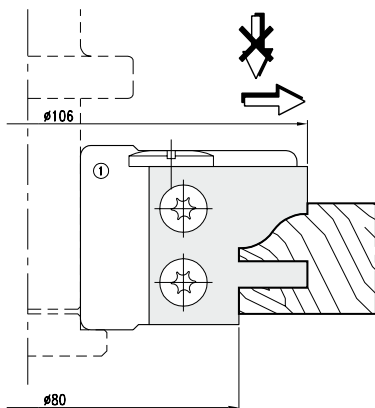
HW Konterprofilfräser Z=2 TC Counterprofile cutter Z=2
