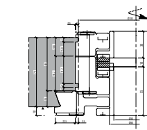
Flügel-Konterprofil N78 Konterprofilierung
