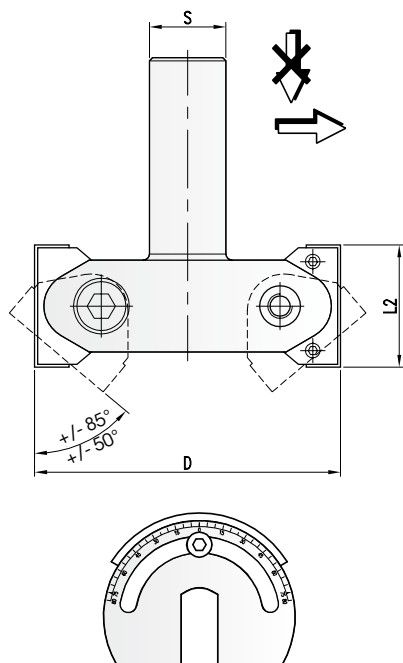
Art.726.102 - Einstelllehre, Skala mit 1° Markierung
