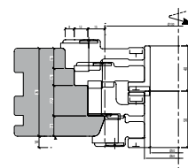
Oberes Blendrahmenholz N78 Doppelkammerprofilierung
