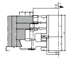
Flüster-Konterprofil N78 Konterprofilierung
