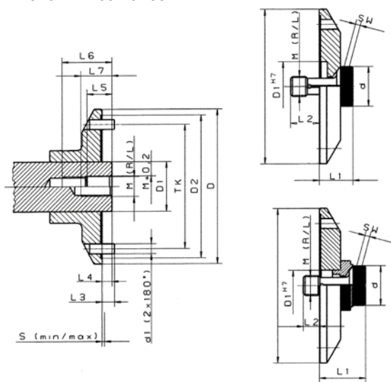
Ausführung A ohne Einsatz Version A without insert
