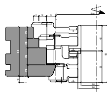
Oberes Blendrahmenholz N/78 Doppelflügelprofilierung
