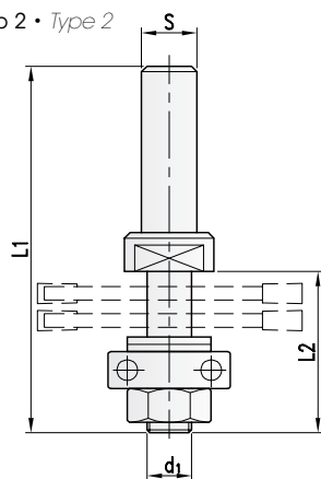
Typ 2 • Type 2
