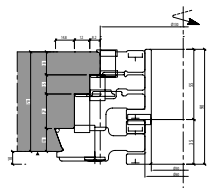
Flüsten-Kontersprofil N/78 Kontersprofilierung
