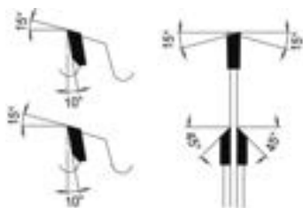
Wechselzahn, Zahn einseitig spitz/plan
