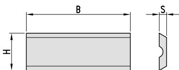
Ausführung 3 - Type 3
