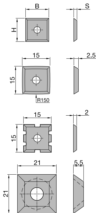
Ausführung 1 - Type 1
