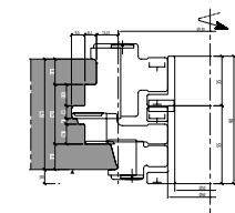
Vertikalfüßchen-Blendrahmen N/78 Kontersprofilierung
