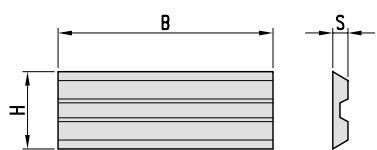
Ausführung 1 - Type 1
