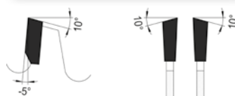
Wechselzahn neg. Spanwinkel
