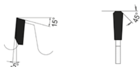
Trapezzahn negativer Spanwinkel
