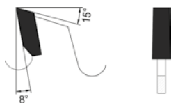
Flachzahn konisch Flat tooth conical
