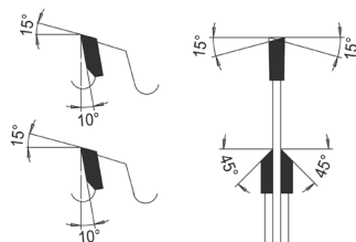
Wechselzahn, Zahn einseitig spitz/plan
