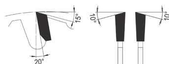
Wechselzahn spandickenbegrenzt Alternate Top Bevel tooth with limited chip thickness
