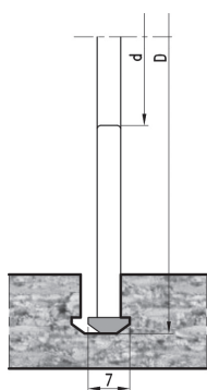
▲ Profilfräsausführung für Lamello® Zeta ▲ profile cutter design for Lamello® Zeta
