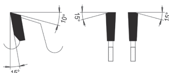
Flachzahn mit wechselseitiger Fase
