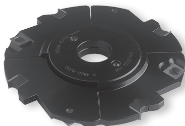
WP-Nutfräsersatz für Handvorschub mit Zwischenringen verstellbar
