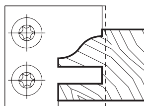
Profilierungsbeispiele profiling examples
