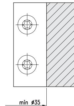
Profilierungsbeispiele profiling examples
