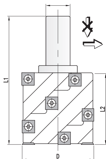
HW-Spiralfräser TC spiral cutter
