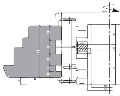
Flügel-Konterprofil IV78 Konterprofilierung sash counter profile IV78 counter-profiling
