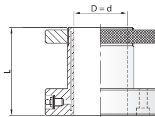
Hydrogrip-Schraubbuchse für Nut- und Federwerkzeuge hydro-grip screw bushing for groove-and-tongue tools
