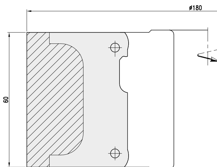
Blankett mit 2-Punkt Auflage blank knife with 2-point support
