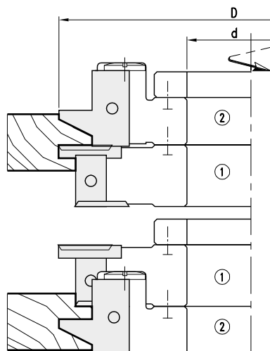
Wechselmesser/Ersatzteile Replacement knives/Spare parts
