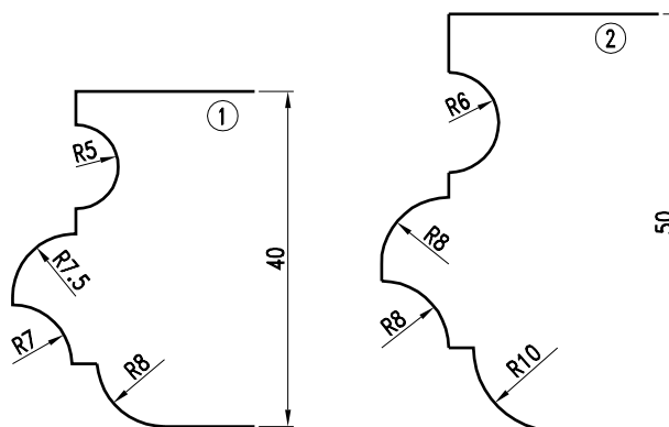
Profilbeispiel example profile
