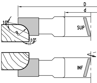
Mit ziehendem Schnitt with axial angle
