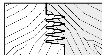
Profilbeispiel Doppelspindelbearbeitung für Holzstärke 18-30mm, Zinkenprofil 10/11 profile example for double-spindle machining for wood thickness 18 to 30 mm, finger joint profile 10/11
