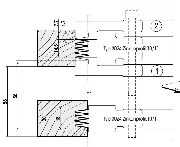
Profilbeispiel Einspindelbearbeitung für Holzstärke 18-30 mm, Zinkenprofil 10/11 profile example for single-spindle machining for wood thickness 18 to 30 mm, finger joint profile 10/11
