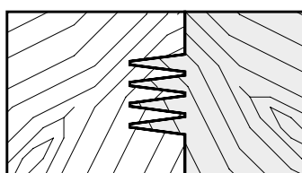
Profilbeispiel Doppelspindelbearbeitung für Holzstärke 18-30mm, Zinkenprofil 10/11 profile example for double-spindle machining for wood thickness 18 to 30 mm, finger joint profile 10/11
