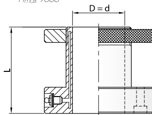
Hydrogrip-Schraubbuchse für Nut- und Federwerkzeuge hydro-grip screw bushing for tongue-and-groove tools
