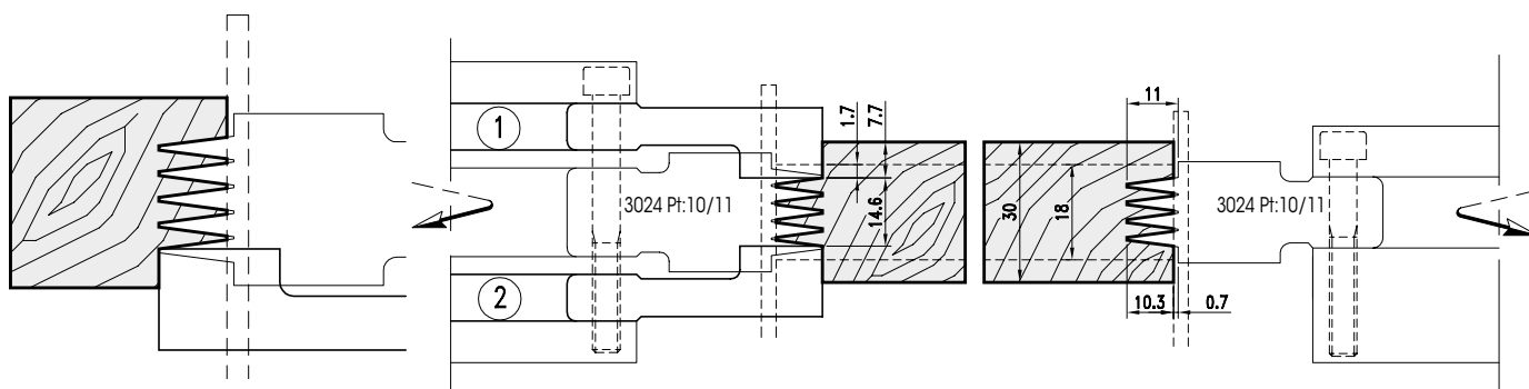
Profilbeispiel Doppelspindelbearbeitung für Holzstärke 18-30mm, Zinkenprofil 10/11 profile example for double-spindle machining for wood thickness 18 to 30 mm, finger joint profile 10/11
