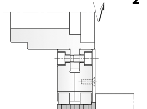
Platte zerspanen und damit untere Deckschicht freilegen Milling panel to uncover lower surface layer
