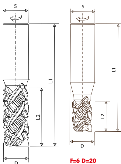
PKD-Schaftfräser mit Z=3+3 PCD shank milling cutter with Z=3+3
