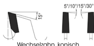
Wechselzahn, konisch
