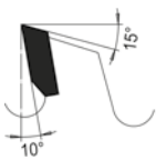
Trapez-Flachzahn
