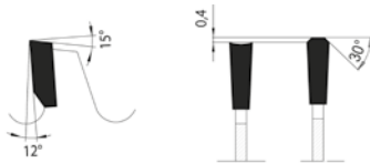
Hohlzahn-Dach-Flach
