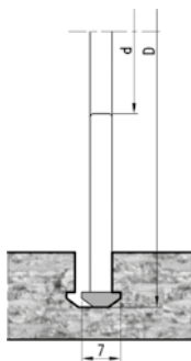
Profilfräsausführung „P“ für Lamello® Zeta Profile cutter design "P" for Lamello® Zeta
