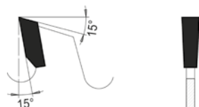
Flachzahn
