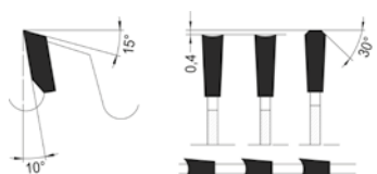
Hohl-Flach-Flach-Trapezzahn
