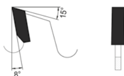
Flachzahn, konisch Flat Top Grind tooth, conical
