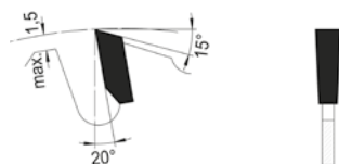
Flachzahn, spandickenbegrenzt
