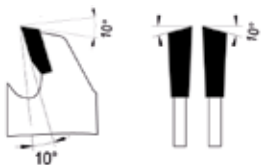
Wechselachzahn Alternate inverted V tooth
