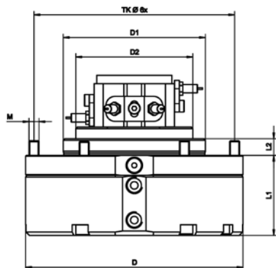
Pneumatische Löseeinheit mit digitaler Sensorik Pneumatic release unit with digital sensors
